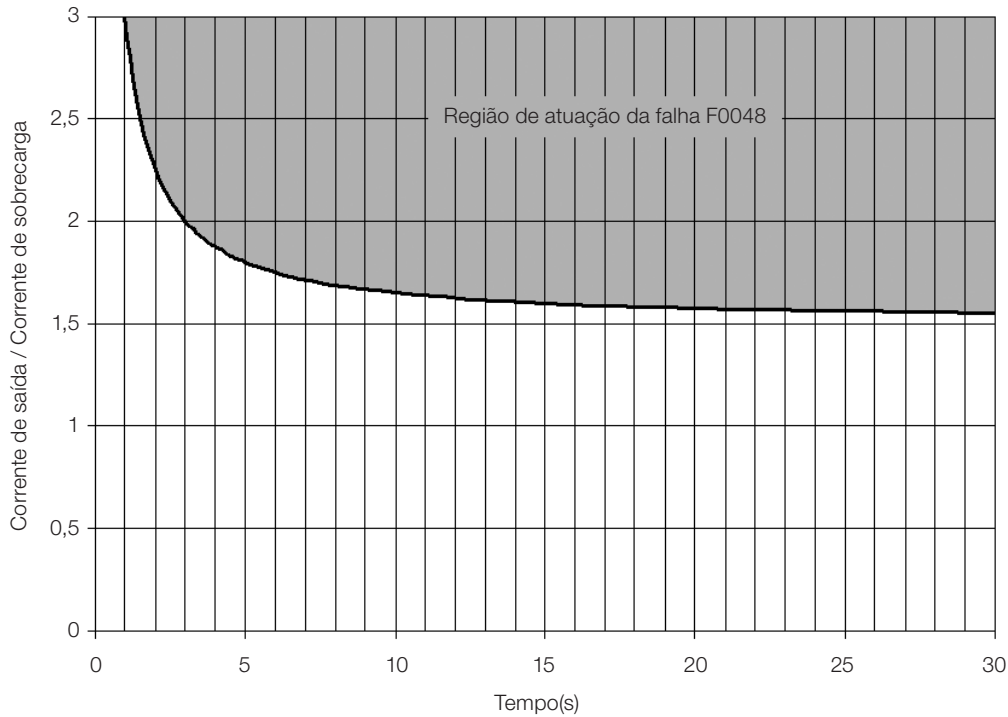
Figura 17.2: Atuação da sobrecarga dos IGBTs
