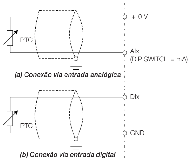
Figura 17.3: (a) e (b) Conexão do PTC ao CFW500
