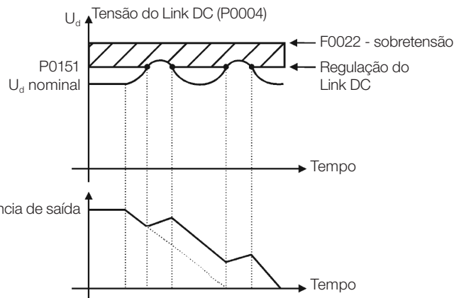
Figura 9.9: Gráfico exemplo da limitação da tensão do Link DC - Acelera Rampa
