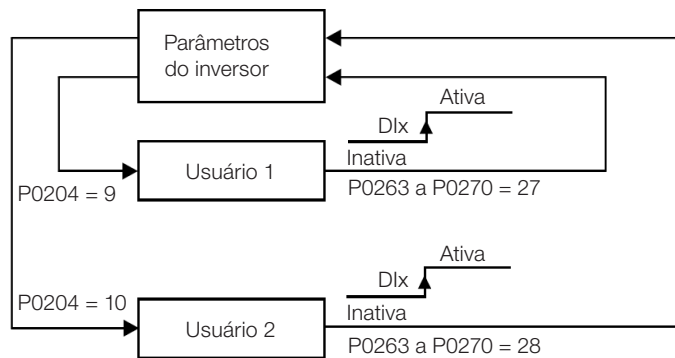
Figura 14.15: Diagrama de blocos das funções carrega us. 1 e us. 2
